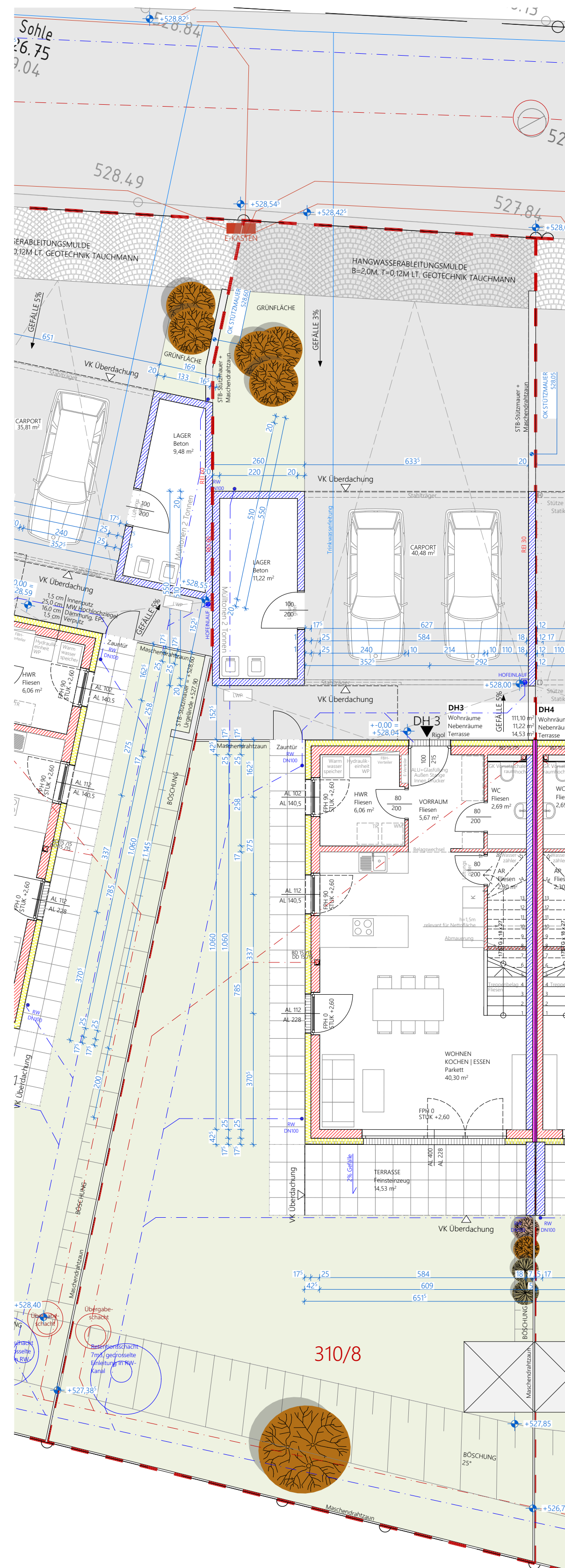
GRUNDRISS ERDGESCHOSS
