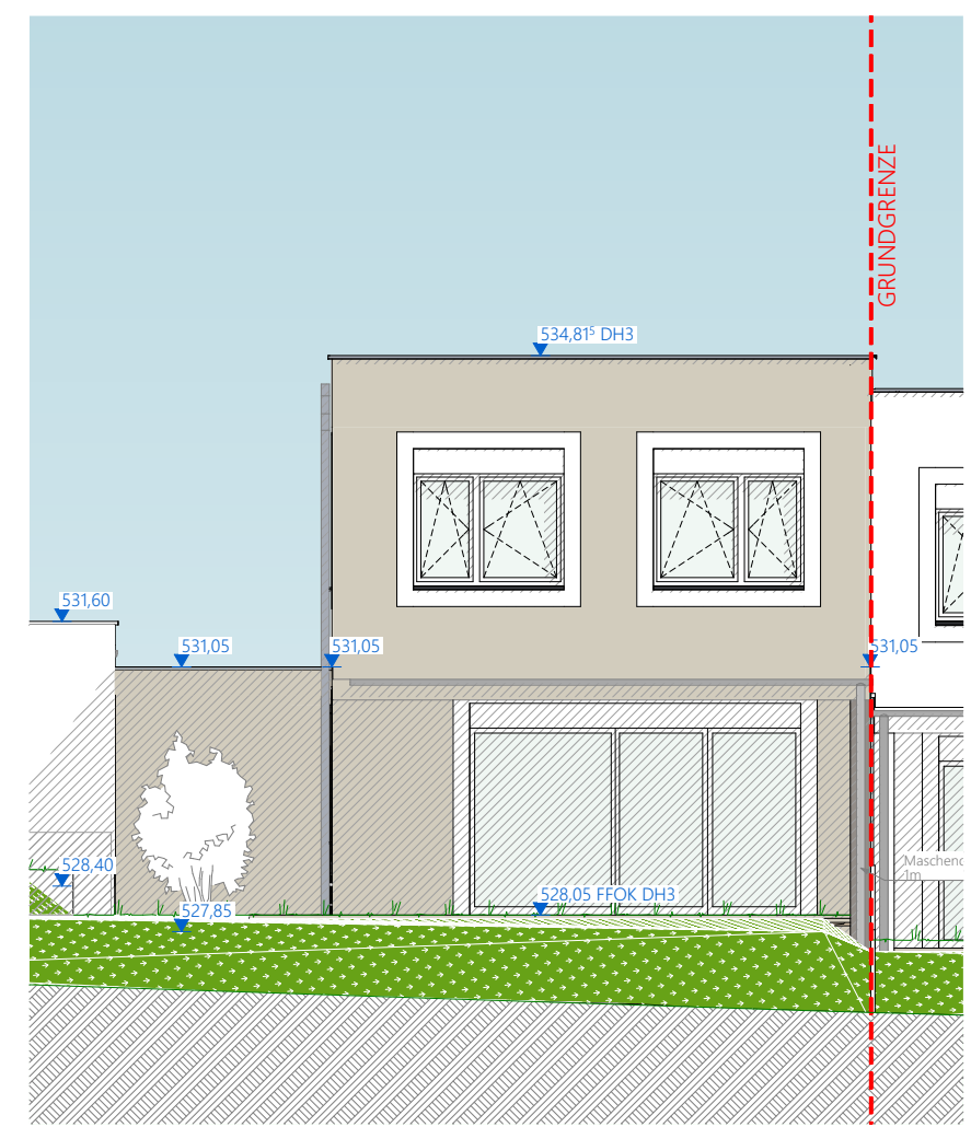
ANSICHT SÜD
